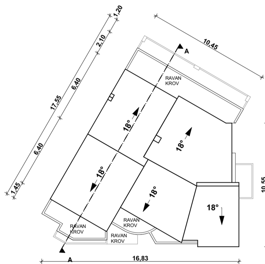
TLOCRT KROVA MJ 1:200
