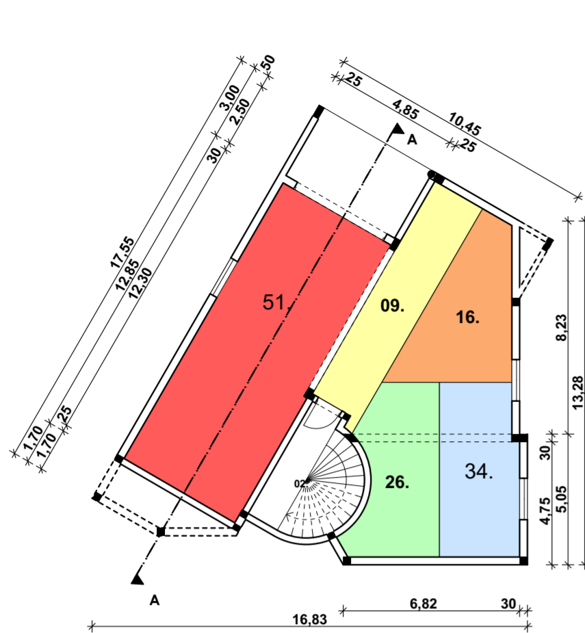
TLOCRT PODRUMA MJ 1:200
