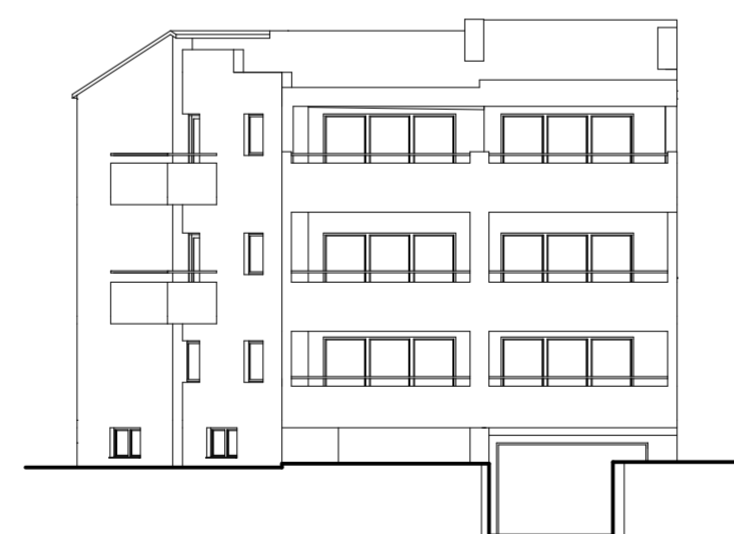
SJEVEROZAPADNO PROČELJE MJ 1:200
