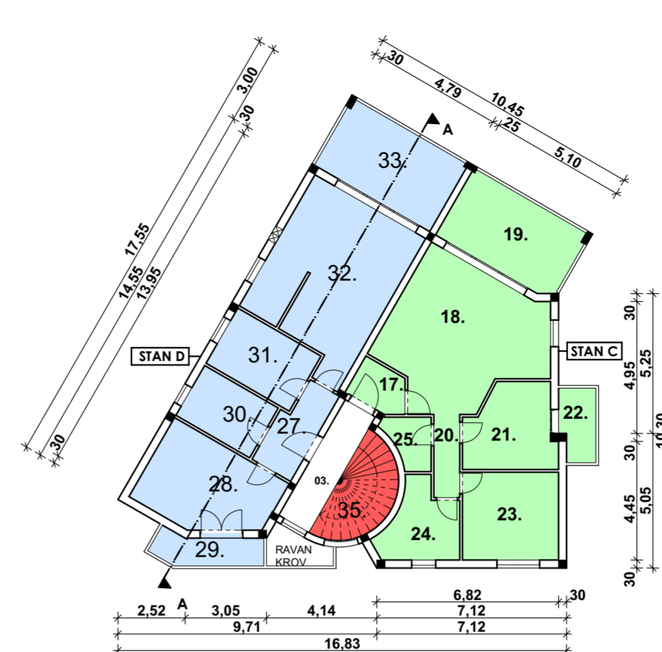
TLOCRT 1. KATA MJ 1:200
