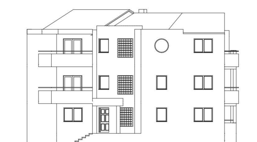
ISTOČNO PROČELJE MJ 1:200
