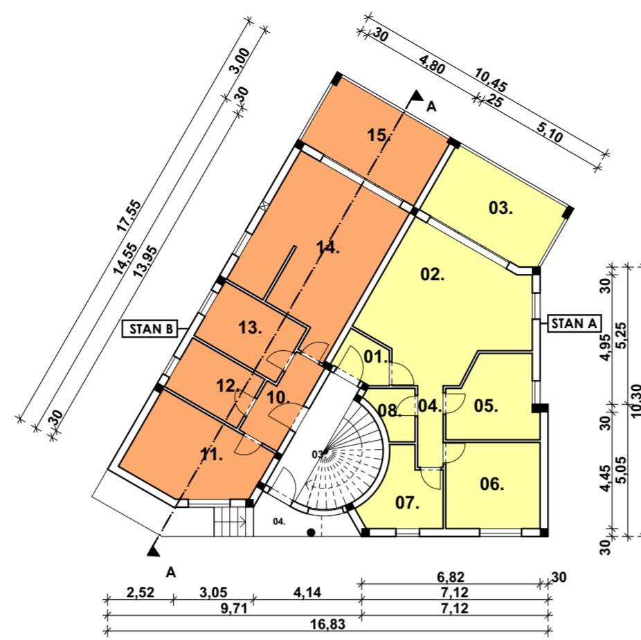
TLOCRT PRIZEMLJA MJ 1:200
