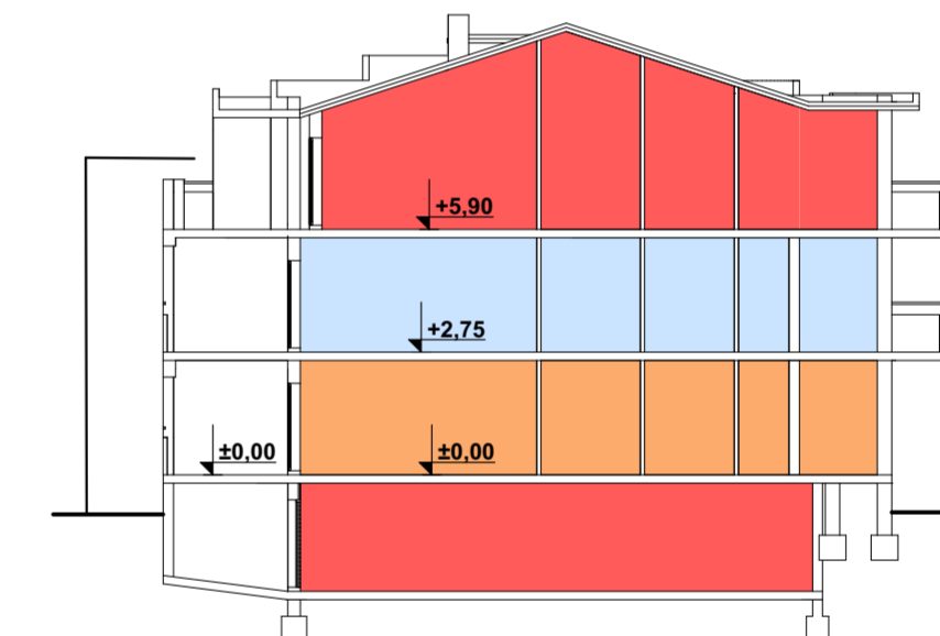
A-A PRESJEK MJ 1:200
