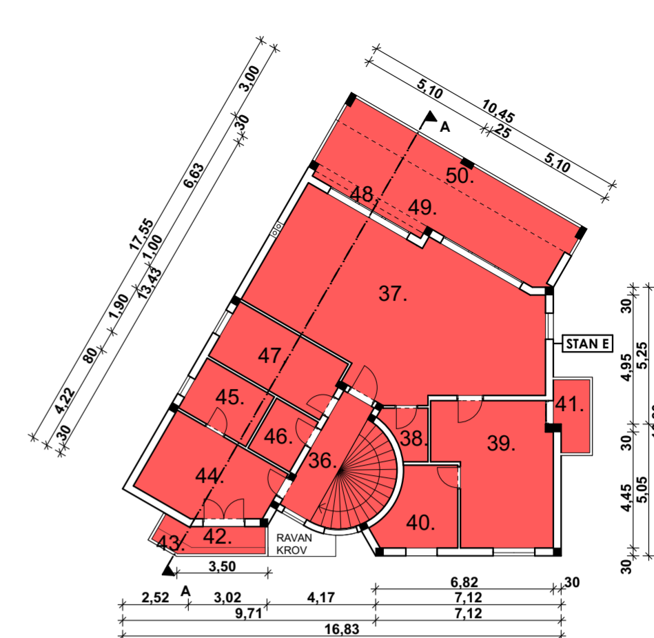
TLOCRT POTKROVLJA MJ 1:200
